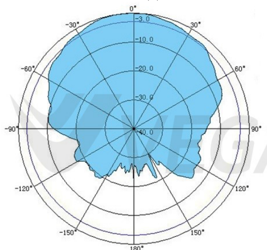
ГОРИЗОНТАЛЬНАЯ ПЛОСКОСТЬ
