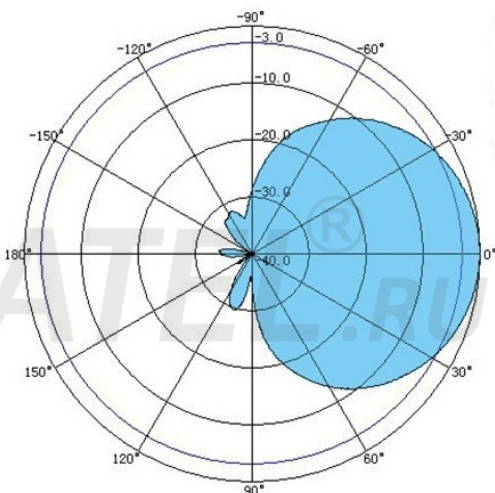
ВЕРТИКАЛЬНАЯ ПЛОСКОСТЬ
